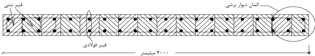
شکل (۲): تقسیم‌بندی مقطع عرضی دیوار به المان فیبر.
